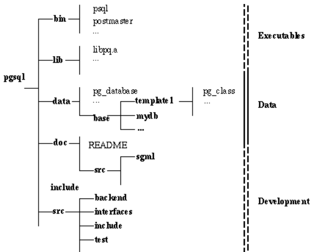
图 19.1. Postgres 文件布局
