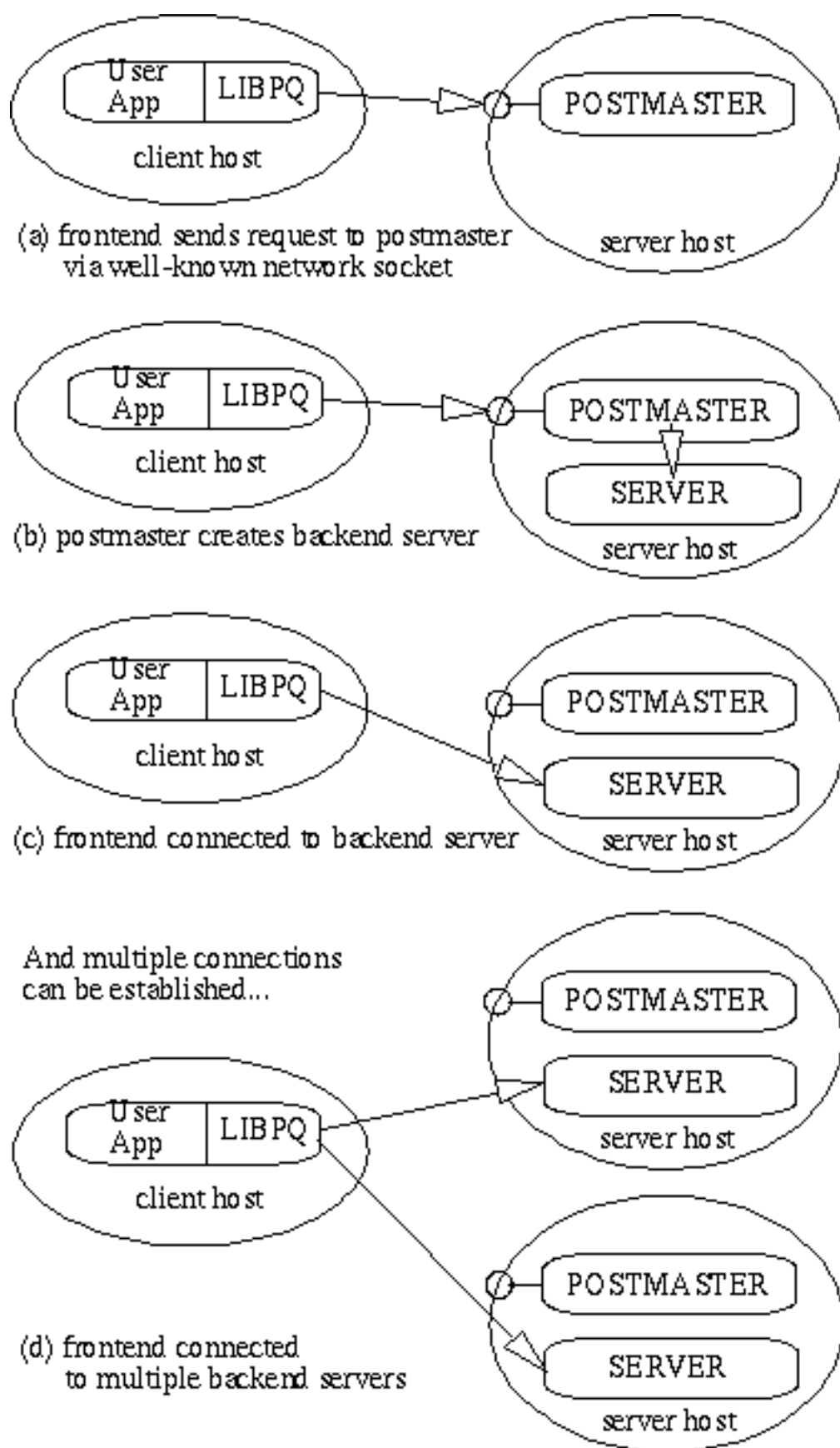
图 29.1. 如何建立连接
