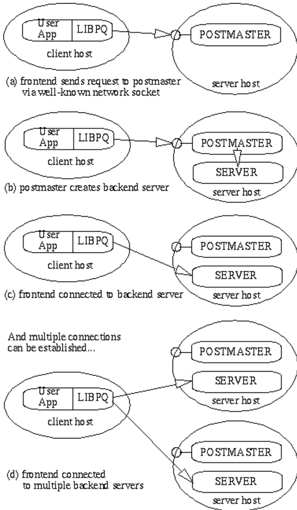
图 49.1. 连接是如何建立的
